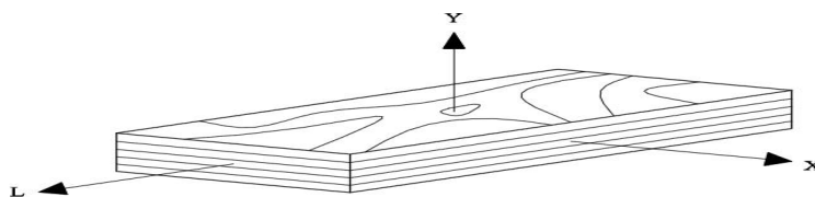
图1 结构用木质材料的方向性
