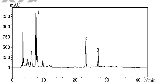
图 B.2 漆树提取物的高效液相色谱图
