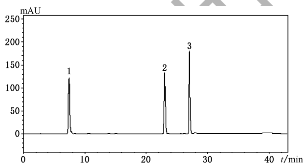
图 B.1 标准样品的高效液相色谱图
